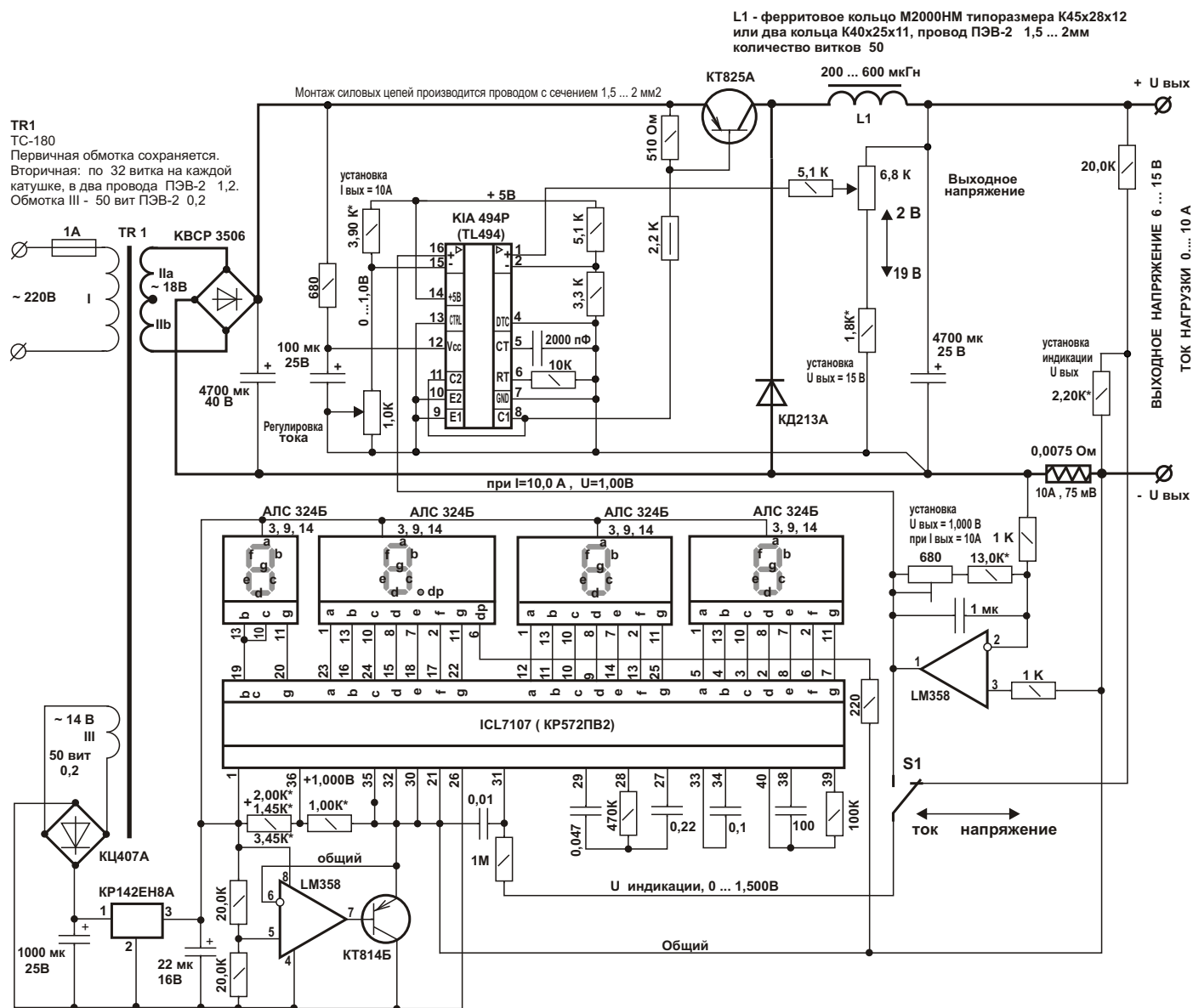
ПРИНЦИПИАЛЬНАЯ СХЕМА ЗАРЯДНОГО УСТРОЙСТВА ДЛЯ АВТОМОБИЛЬНЫХ АККУМУЛЯТОРОВ С ЦИФРОВОЙ ИНДИКАЦИЕЙ ТОКА И НАПРЯЖЕНИЯ
