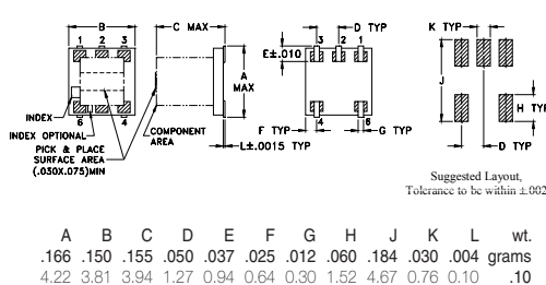
AT1029 (SBTC-2-20L+)
