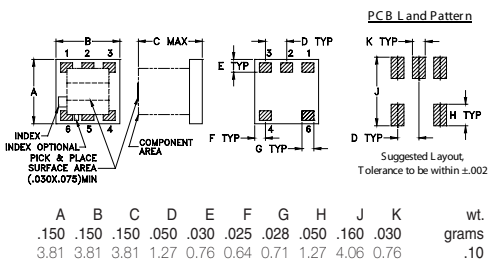
AT790 (SBTC-2-20+)
