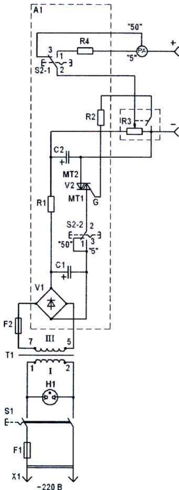
Рисунок 2 - Схема электрическая принципиальная
